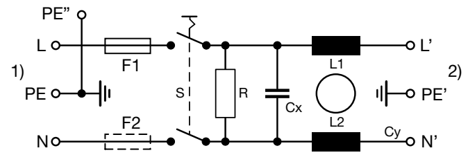
1) Line 2) Load
